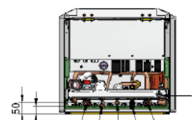
Unteransicht GBK-25C
