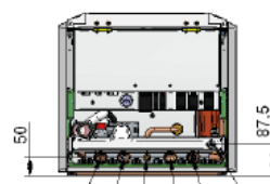
Unteransicht GBK-25 / 35 H/SH
